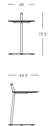
TL-04 Levisium Side Table
